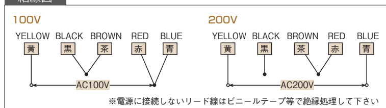
結線図
