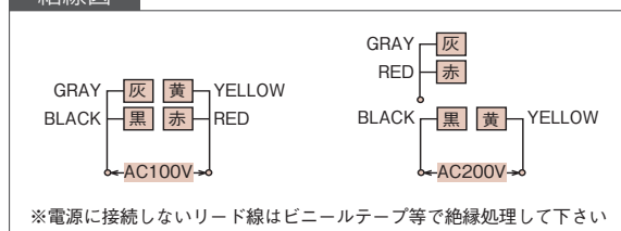
結線図
