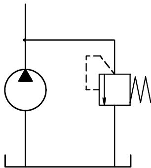
外部リターン式
