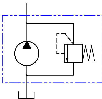
内部リターン式
