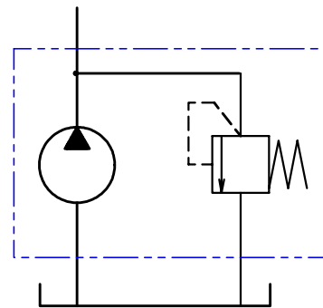
外部リターン式 (2 V D)
