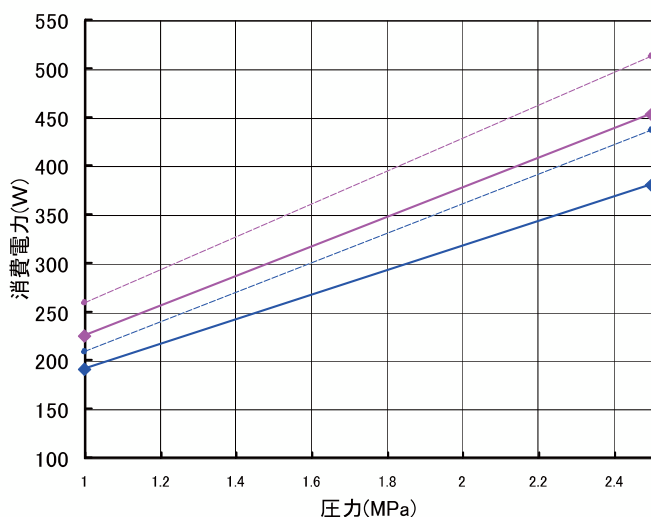
●GFH-V4, V5 消費電力
