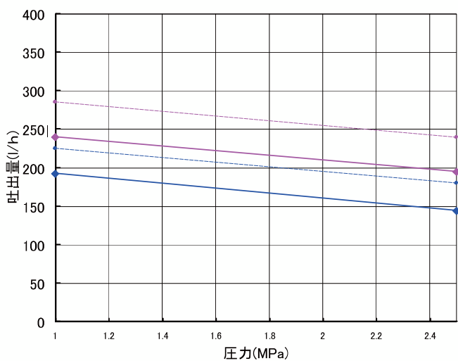
●GFH-V4, V5 吐出量
