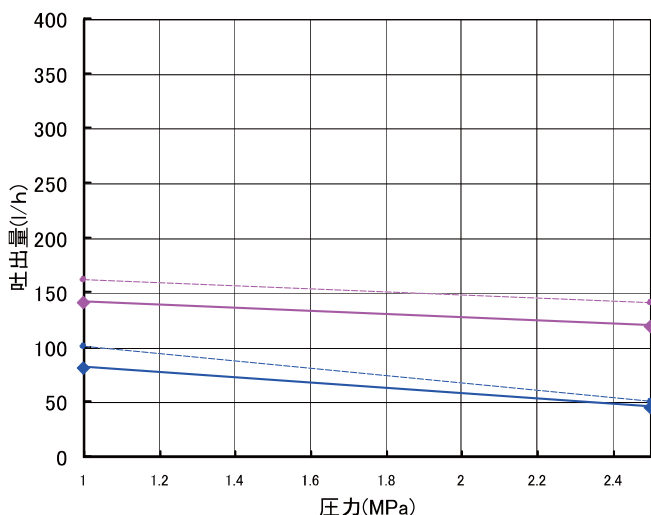
●GFH-V2, V3 吐出量
