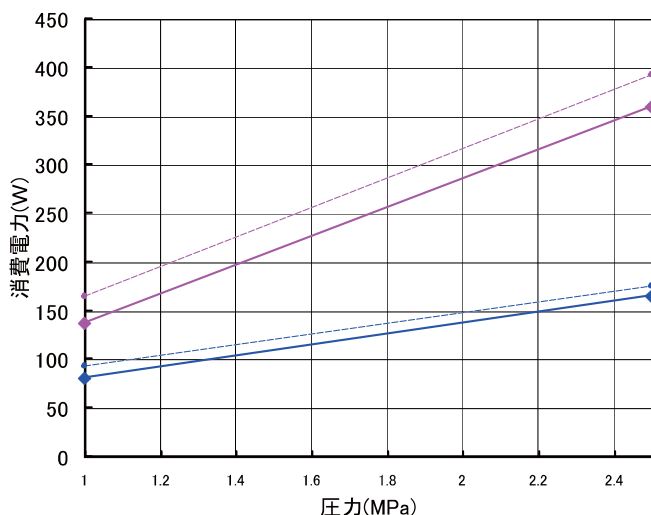
●GFH-V2, V3 消費電力
