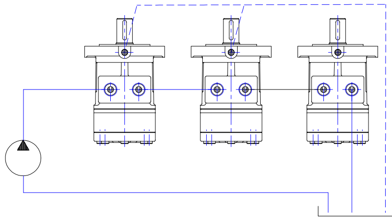
直列接続
