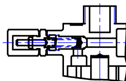
リリーフバルブ詳細
