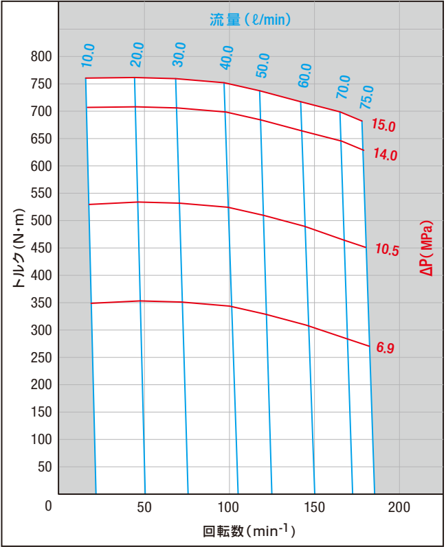
ORB-AH-390
