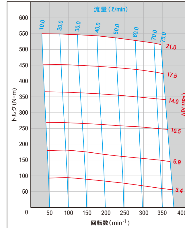
ORB-AH-200
