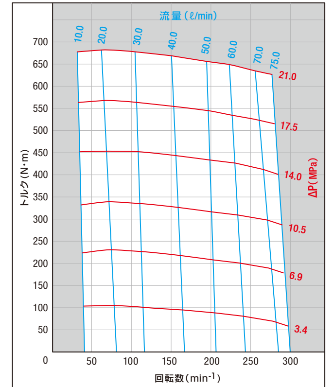
ORB-AH-250
