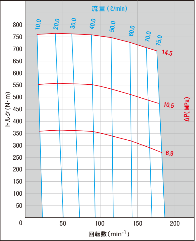
ORB-AH-410
