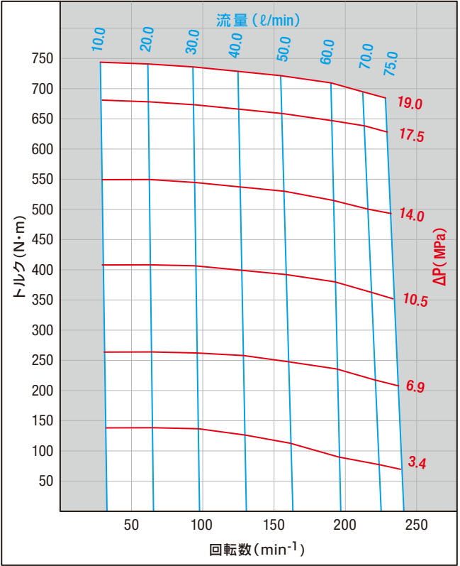
ORB-AH-315
