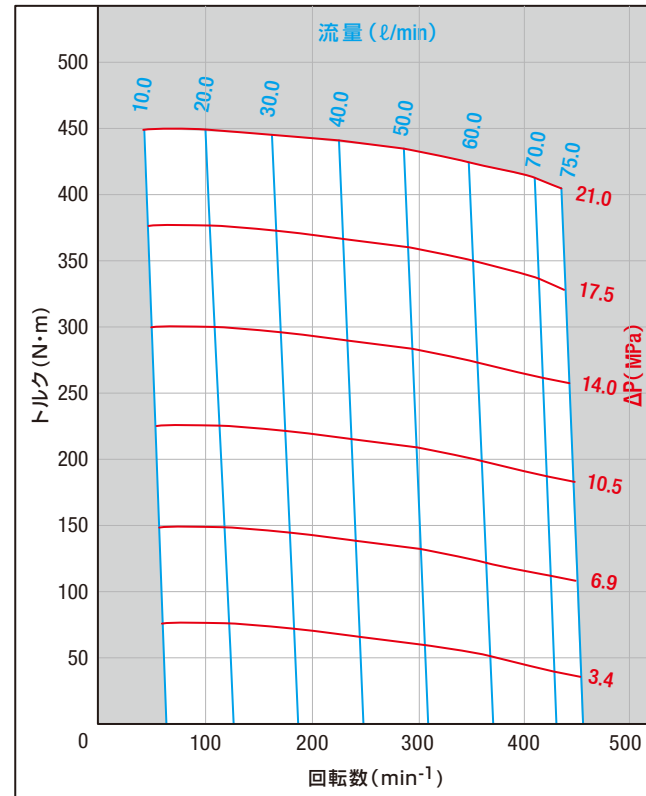
ORB-AH-160
