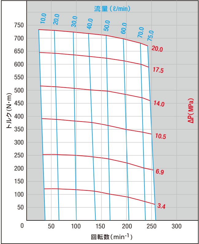
ORB-AH-290
