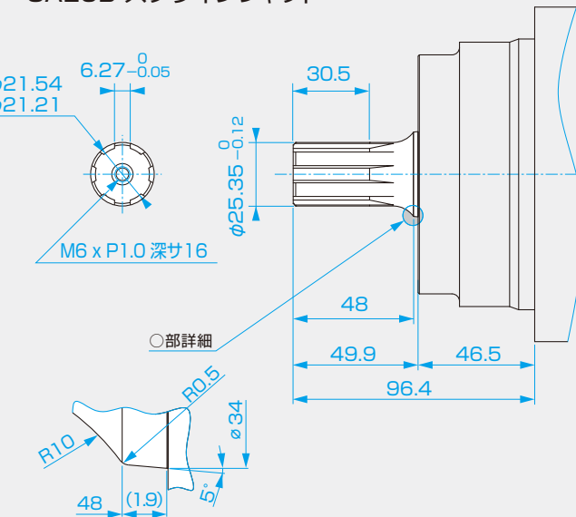
記号 S SAE6B スプラインシャフト
