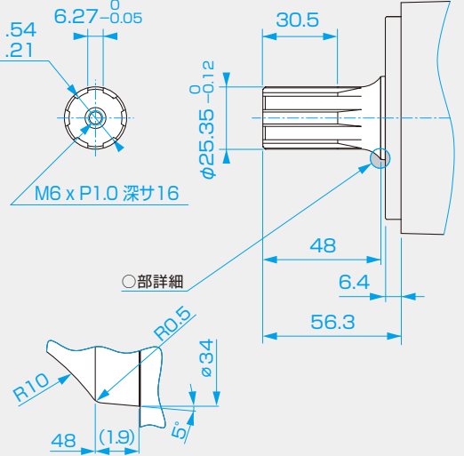
記号 S SAE6B スプラインシャフト
