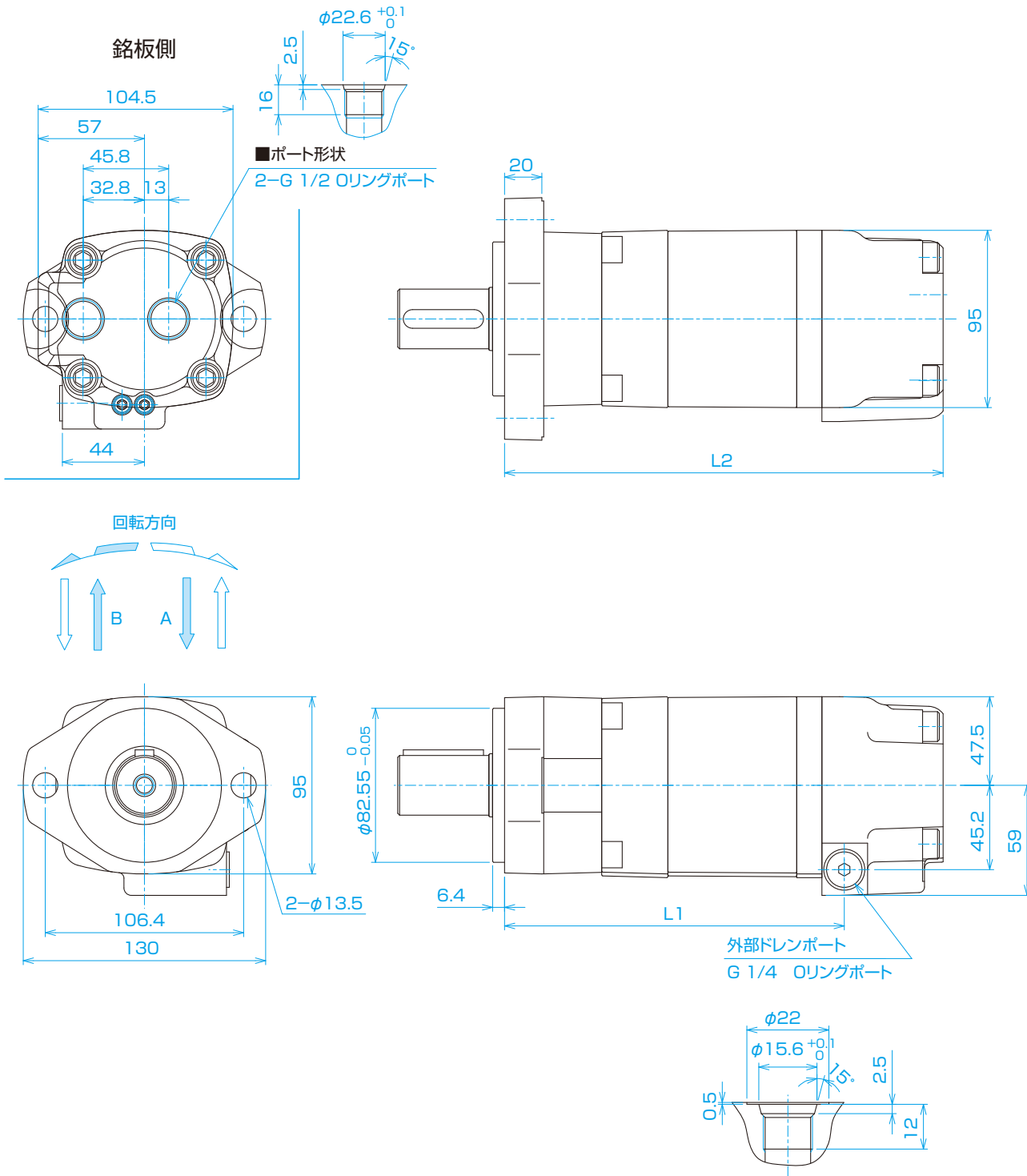
■ 寸法図 ORB-A-***-A*2D
