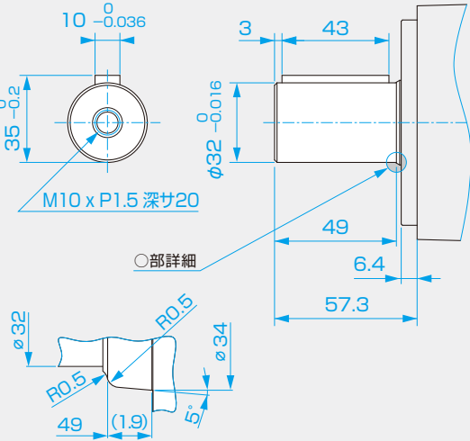
記号 J φ32 シャフト 幅10 キー
