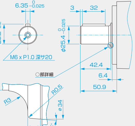
記号 E φ1" シャフト 幅6.35 キー
