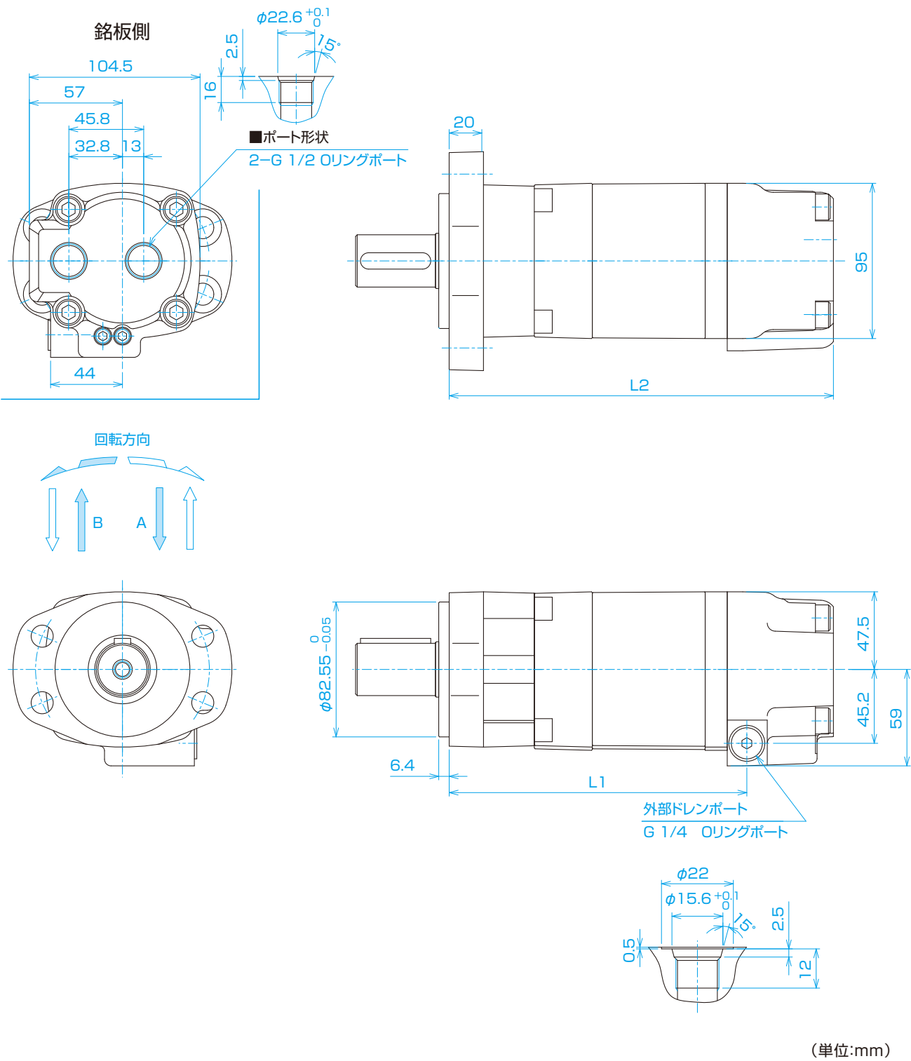
■ 寸法図 ORB-A-***-A*6D
