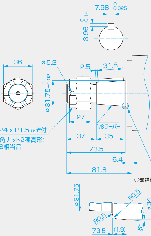
記号 F φ1-1/4" テーパーシャフト(高形ナット) 幅7.96 キー
